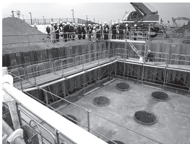
回転圧入鋼管杭（NSエコパイル）工法
