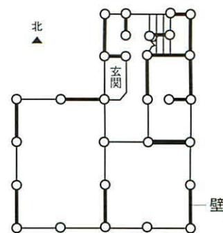
南面に壁がない例
