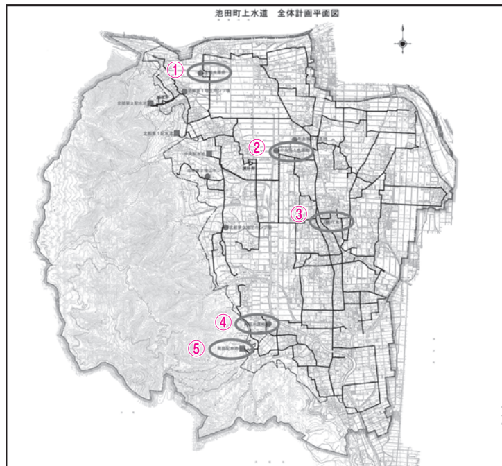
池田町上水道平面図
