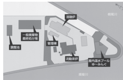
施設配置図
